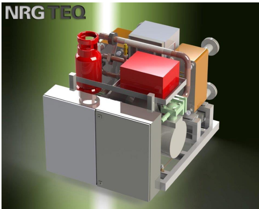
Afpompunit in rood; ingebouwde uitvoering
